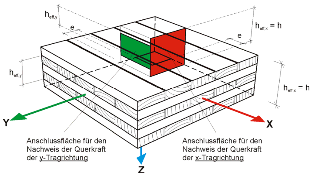
Figure 18: Anschlussflächen für den Nachweis der Querkräfte – beispielhaft für eine Punktlagerung an der Plattenecke
