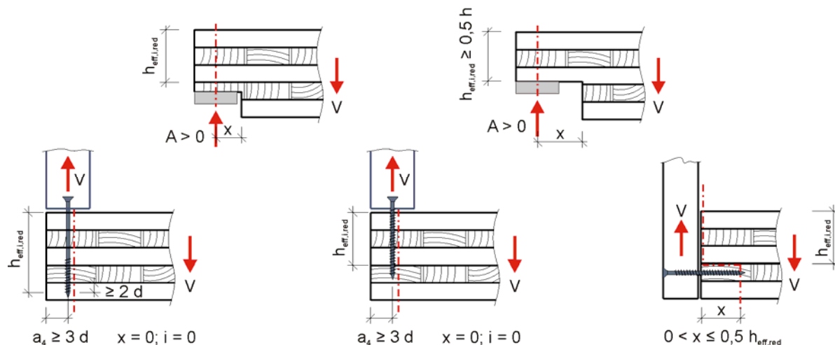
Abbildung 15: Reduzierte Querschnittshöhe, h_{\text{eff}} , zur Berechnung von Ausklinkungen
