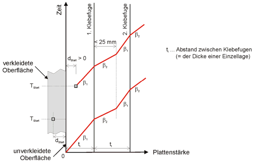
Abbildung 21: Abbrandverhalten mit und ohne Verkleidung
