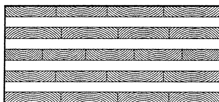
Bild 3: Typische Beispiele für den Aufbau der Massivholzplatte
