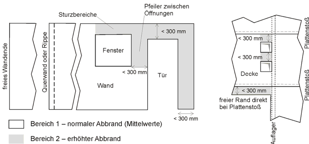
Abbildung 23: Definition von Bereichen für die Bemessung mit normalem oder erhöhtem Abbrand
