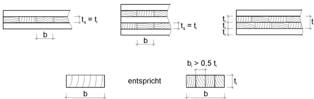
Bild 4: Typische Querschnittsabmessungen von Lamellen für KLH Massivholzplatten
