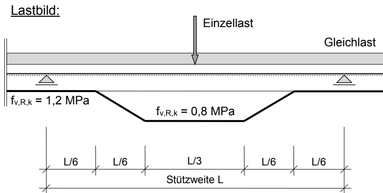
Abbildung 14: Charakteristische Werte der Rollschubfestigkeit für Querkraftanteile infolge Einzellast im Bereich der Feldmitte
