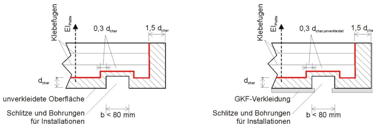
Abbildung 24: Abbrandverhalten im Bereich von Schlitzten und Wandenden
