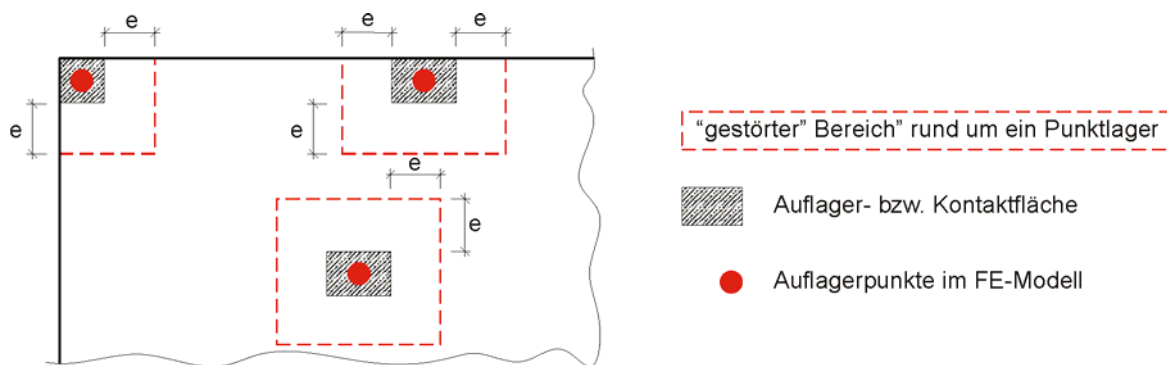
Abbildung 17: Schnittführung rund um Punktlager oder Punktlasten zur Berechnung der Schubspannungen
