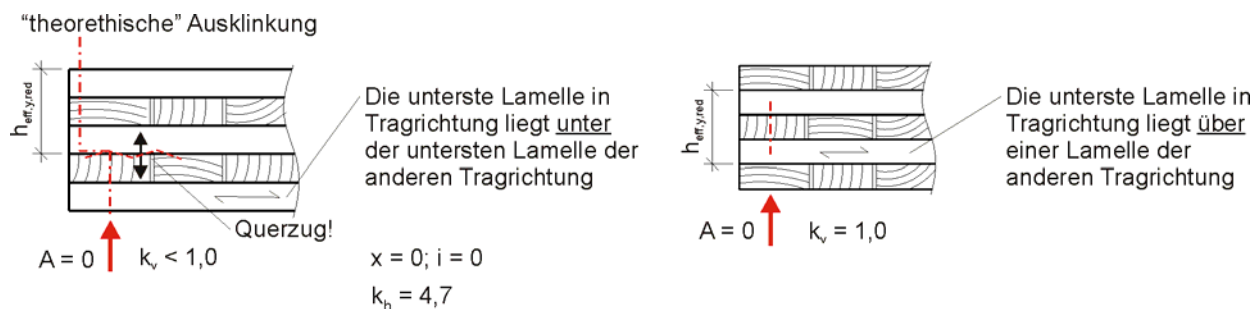
Abbildung 16: Links – teilweise unterstützter Rand – normal zur Deckschicht Rechts – teilweise unterstützter Rand – parallel zur Deckschicht
