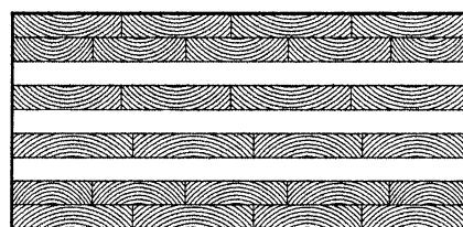
Bild 3: Typische Beispiele für den Aufbau der Massivholzplatte
