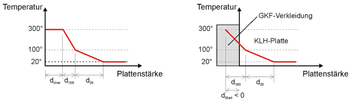
Abbildung 22: Temperaturverlauf für unverkleidete und verkleidete KLH-Massivholzplatten
